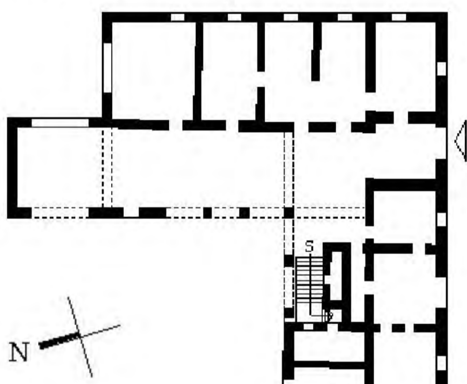
Planta arquitectónica de la casa de la ex hacienda. CNMH-CONACULTA-INAH-MEX.
