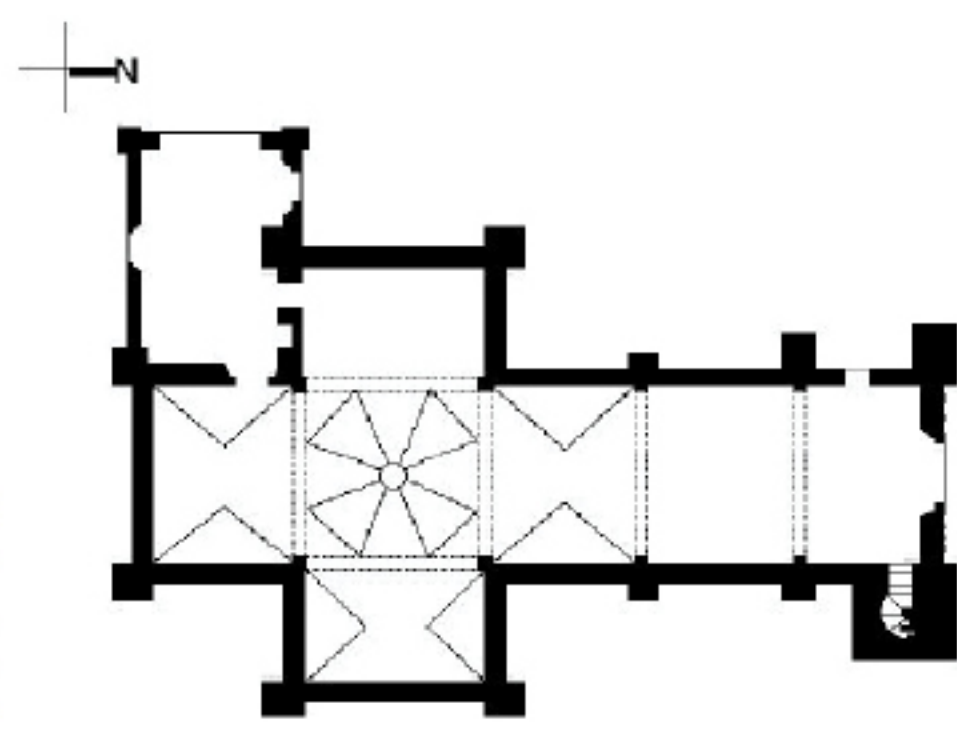
Planta arquitectónica. CNMH-CONACULTA- INAH-MEX.
